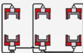
Jeu de 6 colonnes / Satz mit 6 Säulen ERCO-LE -4 + ERCO-LE -2
